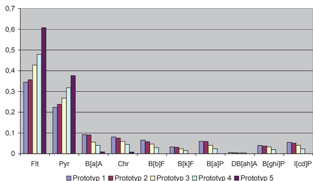
Tabulka 2 Prototypy PAH jaro
