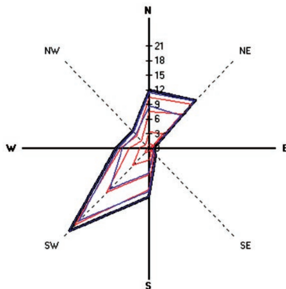
Obrázek 3 Větrná růžice – Ostrava město
