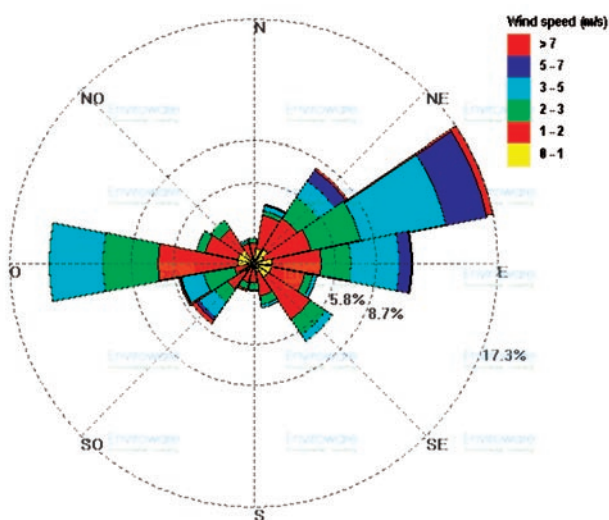
Obrázek 2 Větrná růžice – WindRose
