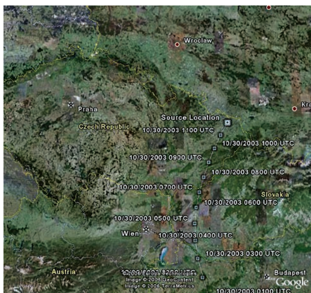
Obrázek 5 HYSPLIT output 30/10/2003 GoogleEarth
