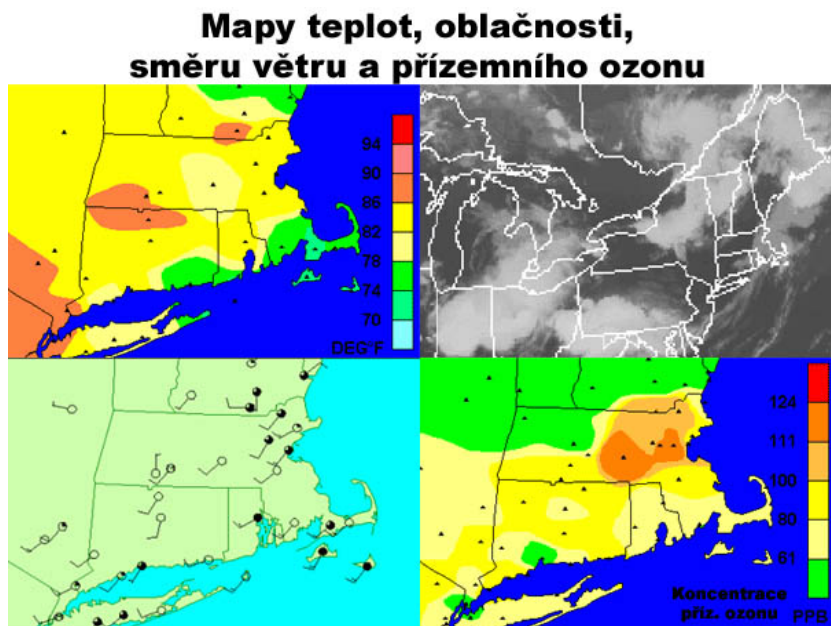
Obr. 1. Ukázka sledování různých parametrů a veličin při vyhodnocování vzniku a koncentrace přízemního ozonu – teploty, směr větru a oblačnost. Pozn.: údaje v PPB převedeme na % obj. vynásobením 10^{-7} .
