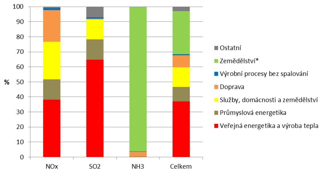
Graf 2 → Zdroje emisí oxyselujících látek v ČR [%], 2012
