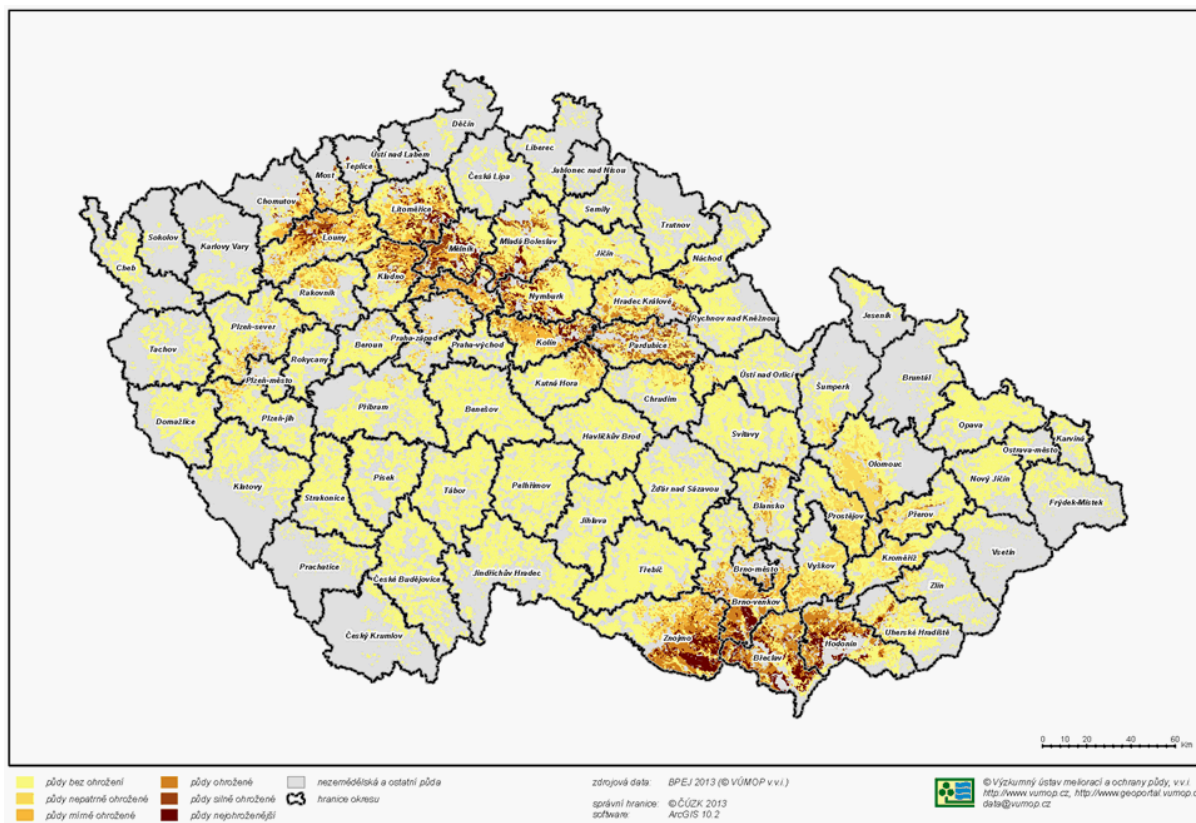
Obr. 3 → Potenciální ohroženost zemědělské půdy větrnou erozí v ČR, 2013
