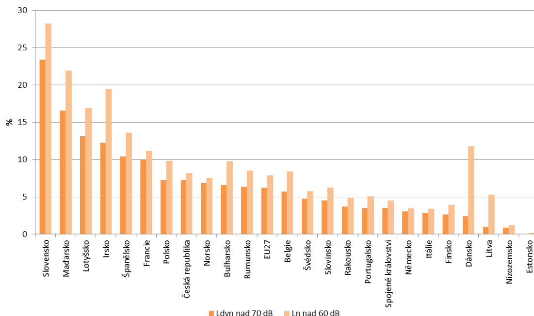
Graf 4 → Hluková zátěž ze silniční dopravy v aglomeracích nad 250 tis. obyvatel, přesahující mezní hodnoty dle legislativy ČR pro celodenní obtěžování hlukem ( L_{dvn} ) a noční hlukovou zátěž ( L_n ) [% exponovaných obyvatel aglomerací], 2009
