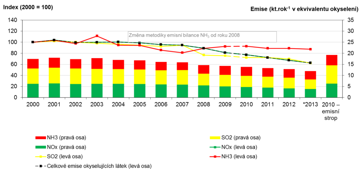
Graf 1 → Vývoj celkových emisí oxyselujících látek v ČR a úroveň národních emisních stropů pro rok 2010 [index, 2000 = 100]; [kt.rok -1 v ekvivalentu oxyselení], 2000–2013
