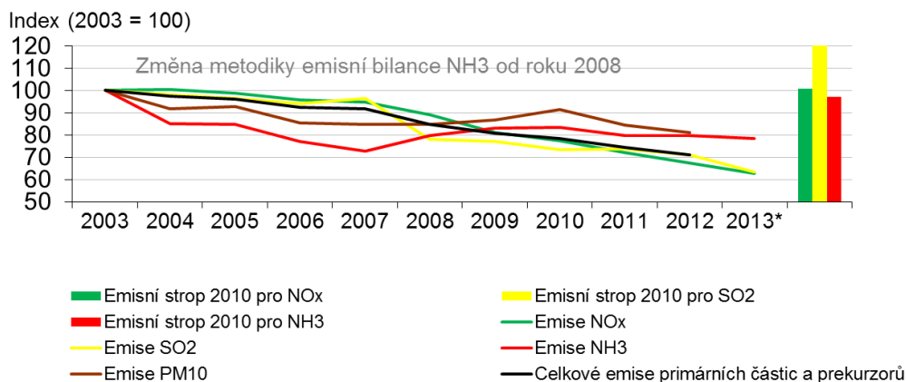
Graf 1 → Vývoj emisí primárních částic a prekurzorů sekundárních částic v ČR a úroveň národních emisních stropů (pro NO x , SO 2 a NH 3 ) pro rok 2010 [index, 2003 = 100], 2003–2013
