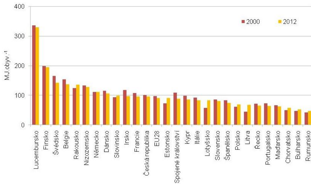
Graf 3 → Konečná spotřeba energie na obyvatele [MJ.obyv. -1 ], 2000, 2012
