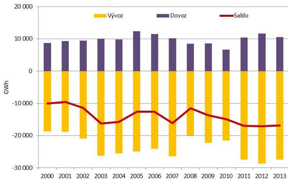
Graf 4 → Dovozy a vývozy elektrické energie v ČR [GWh], 2000–2013
