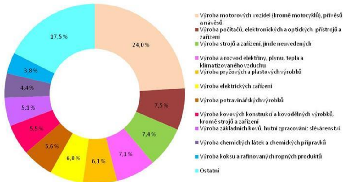
Graf 2 → Struktura průmyslové výroby v ČR [%], 2013
