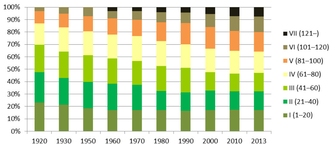
Graf 5 → Vývoj věkové struktury lesních porostů v ČR [%], 1920–2013
