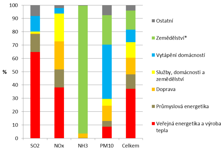
Graf 2 → Zdroje emisí primárních částic a prekurzorů sekundárních částic v ČR [%], 2012
