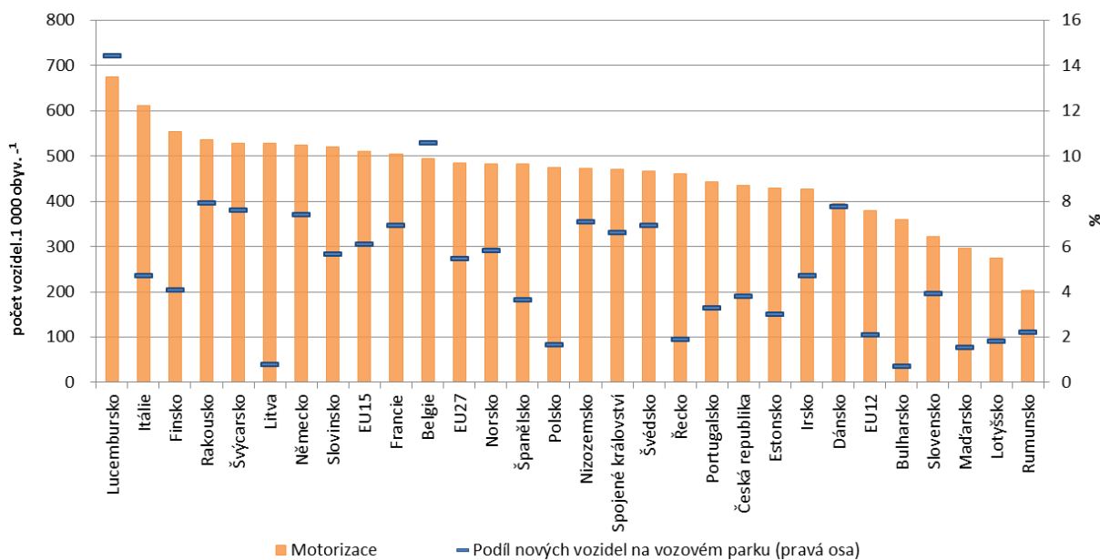
Graf 3 → Motorizace a podíl nových vozidel na celkové velikosti vozového parku osobních automobilů [počet vozidel.1 000 obyv. -1 , %], 2011
