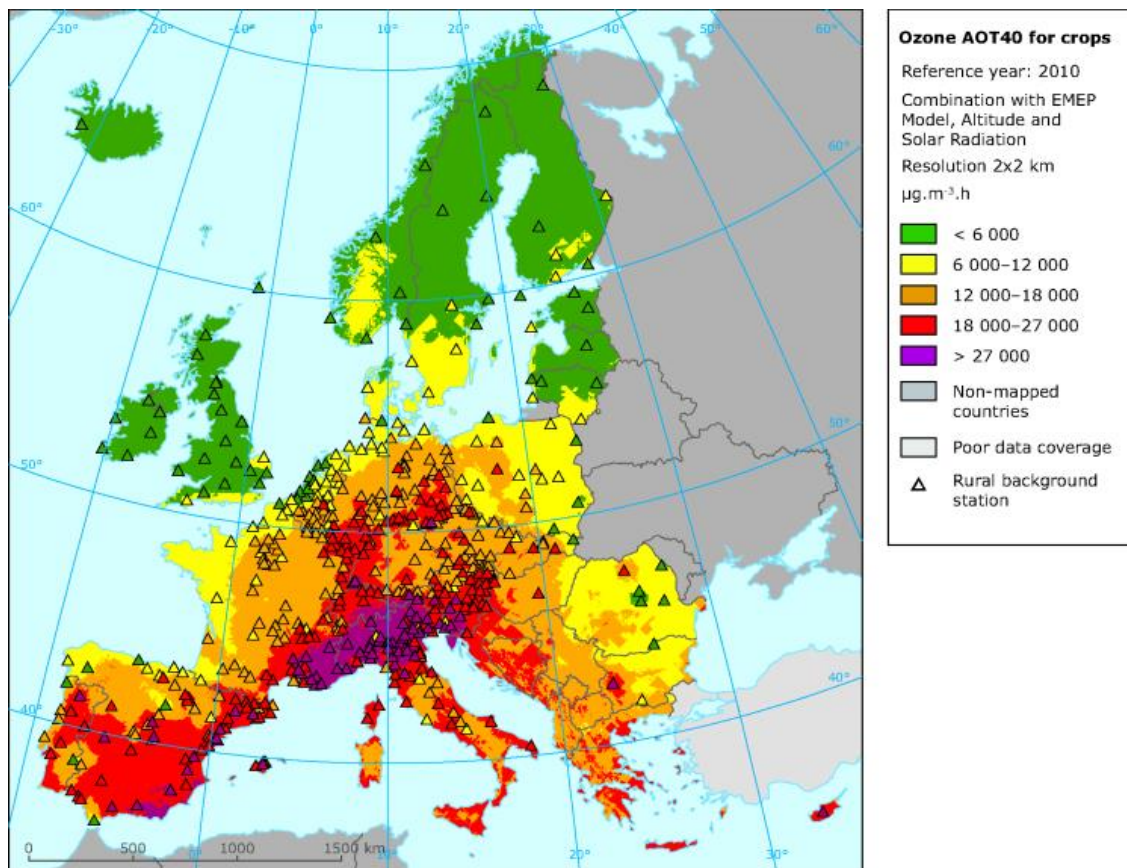
Obr. 1 → Pole hodnot indexu AOT40 v Evropě [ \mu\text{g}\cdot\text{m}^{-3}\cdot\text{h} ], 2010
