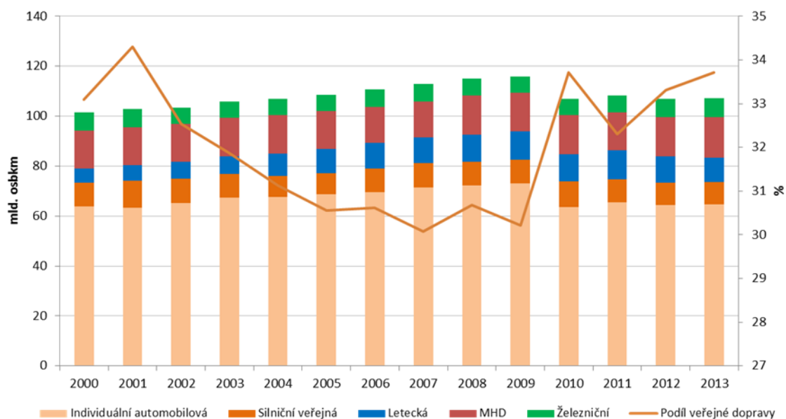
Graf 1 → Vývoj přepravních výkonů osobní dopavy v ČR a podíl veřejné dopavy na osobní dopravě [mld. osbkkm, %], 2000–2013
