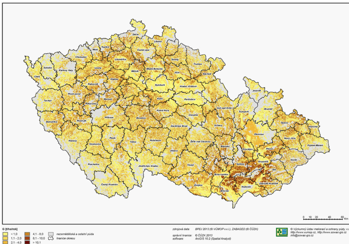
Obr. 1 → Potenciální ohroženost zemědělské půdy vodní erozí v ČR, vyjádřená dlouhodobým průměrným smyvem půdy, 2013
