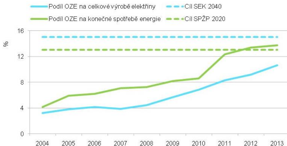
Graf 3 → Cíle pro OZE a stav jejich plnění v ČR [%], 2004–2013
