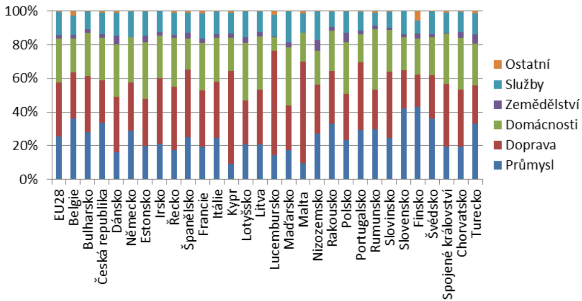
Graf 4 → Konečná spotřeba energie dle sektorů [%], 2012
