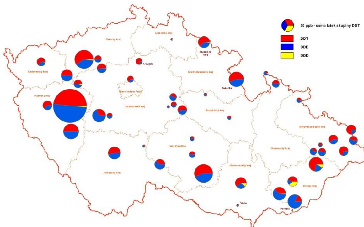
Obr. 1 → Obsah látek skupiny DDT v ornici zemědělských půd v ČR (v rámci Bazálního monitoringu půd) [ \mu\text{g}\cdot\text{kg}^{-1} ], 2013
