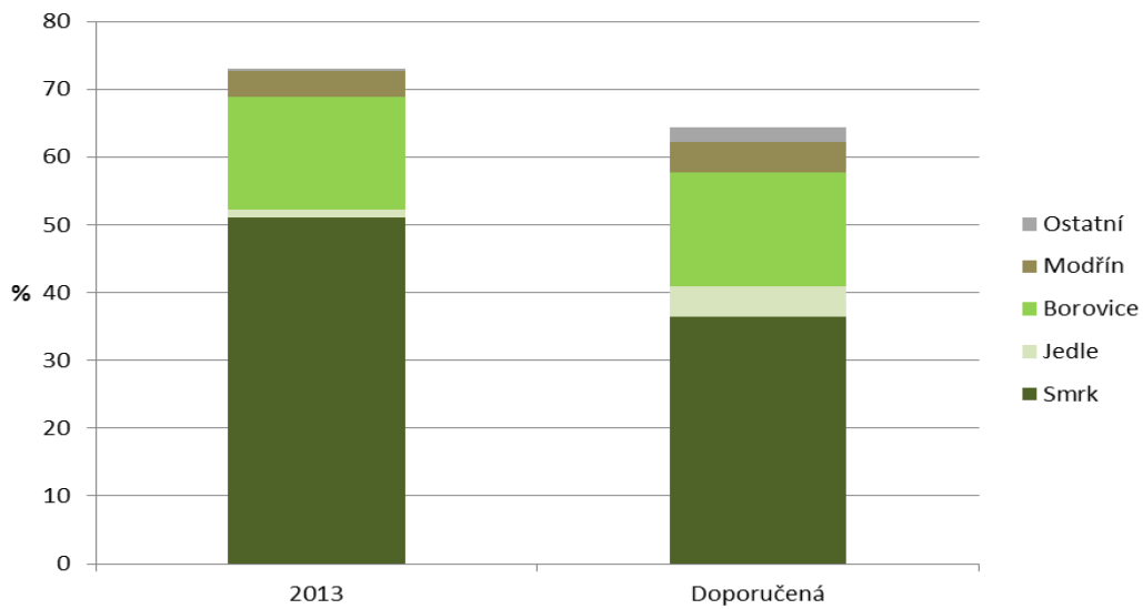
Graf 3 → Současná druhová skladba jehličnatých porostů v ČR v porovnání s doporučenou skladbou [%], 2013
