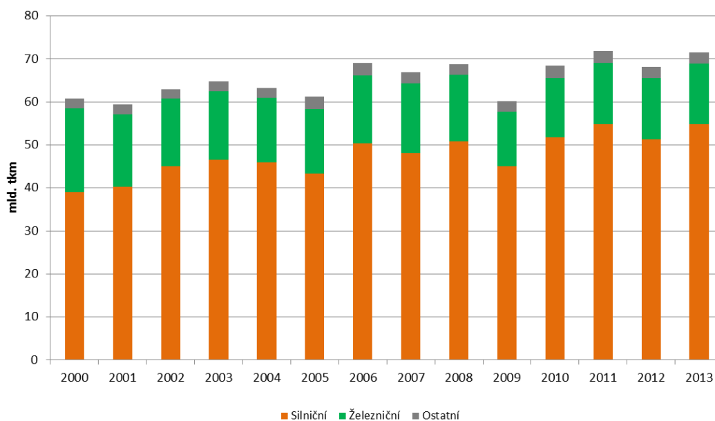
Graf 2 → Vývoj přepravních výkonů nákladní dopavy v ČR [mld. tkm], 2000–2013
