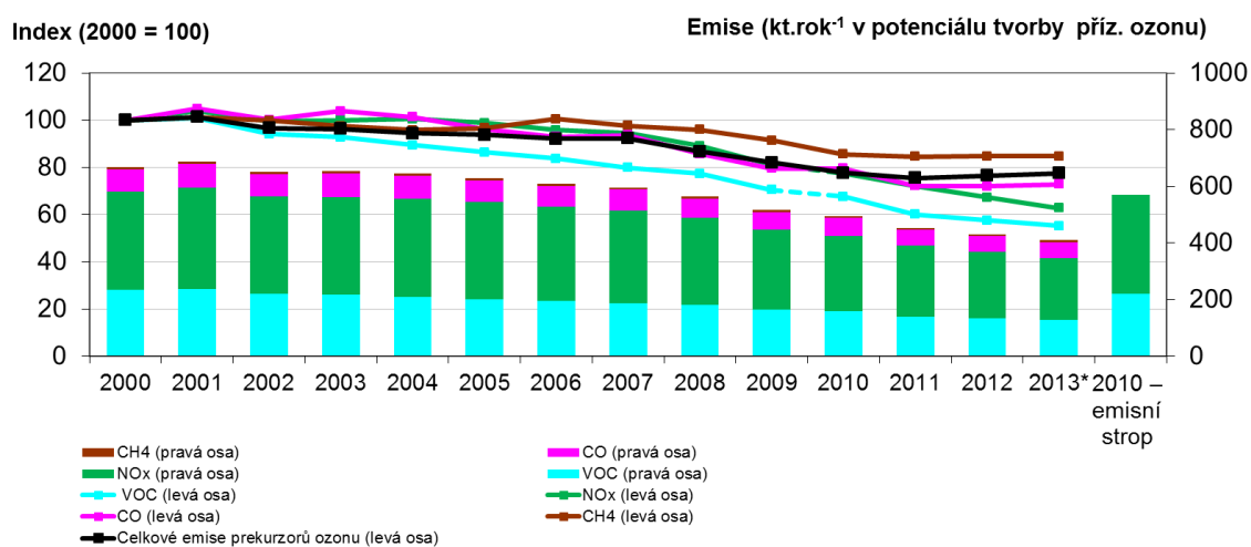
Graf 1 → Vývoj celkových emisí prekurzorů ozonu v ČR a úrovně národních emisních stropů (pro VOC a NO x ) pro rok 2010 [index, 2000 = 100]; [kt.rok -1 v potenciálu tvorby přízemního ozonu], 2000–2013
