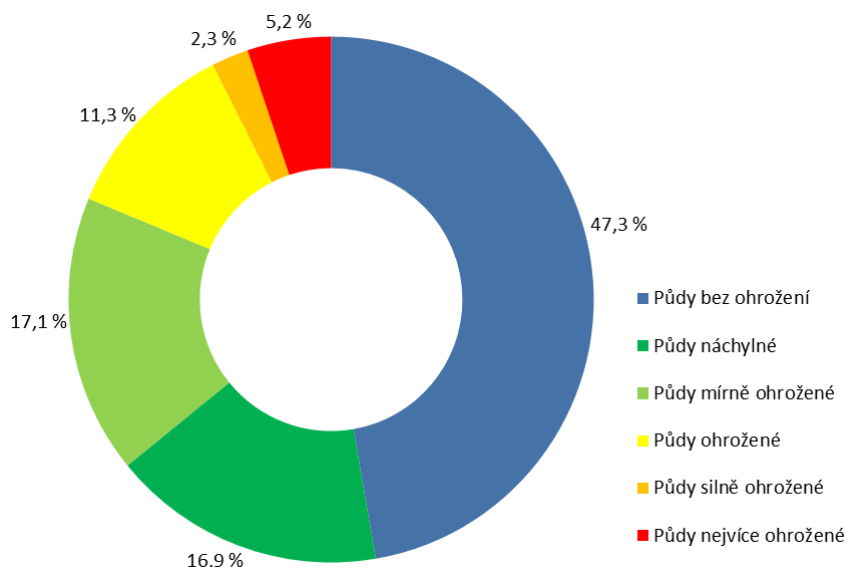
Graf 1 → Potenciální ohroženost zemědělské půdy vodní erozí v ČR, vyjádřená dlouhodobým průměrným smyvem půdy [% ZPF], 2013
