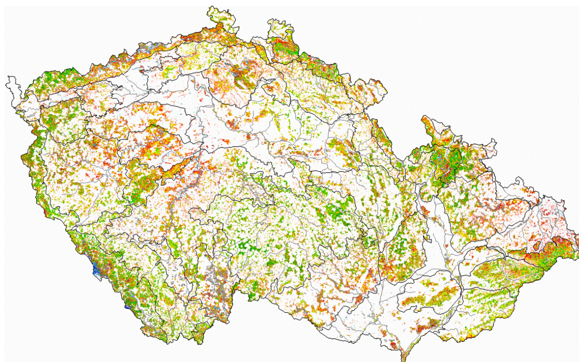
Obr. 1 → Dynamika zdravotního stavu lesních porostů 2001–2012
